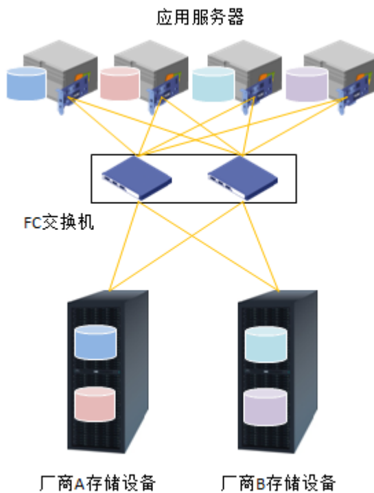
图4-1 原始组网图
