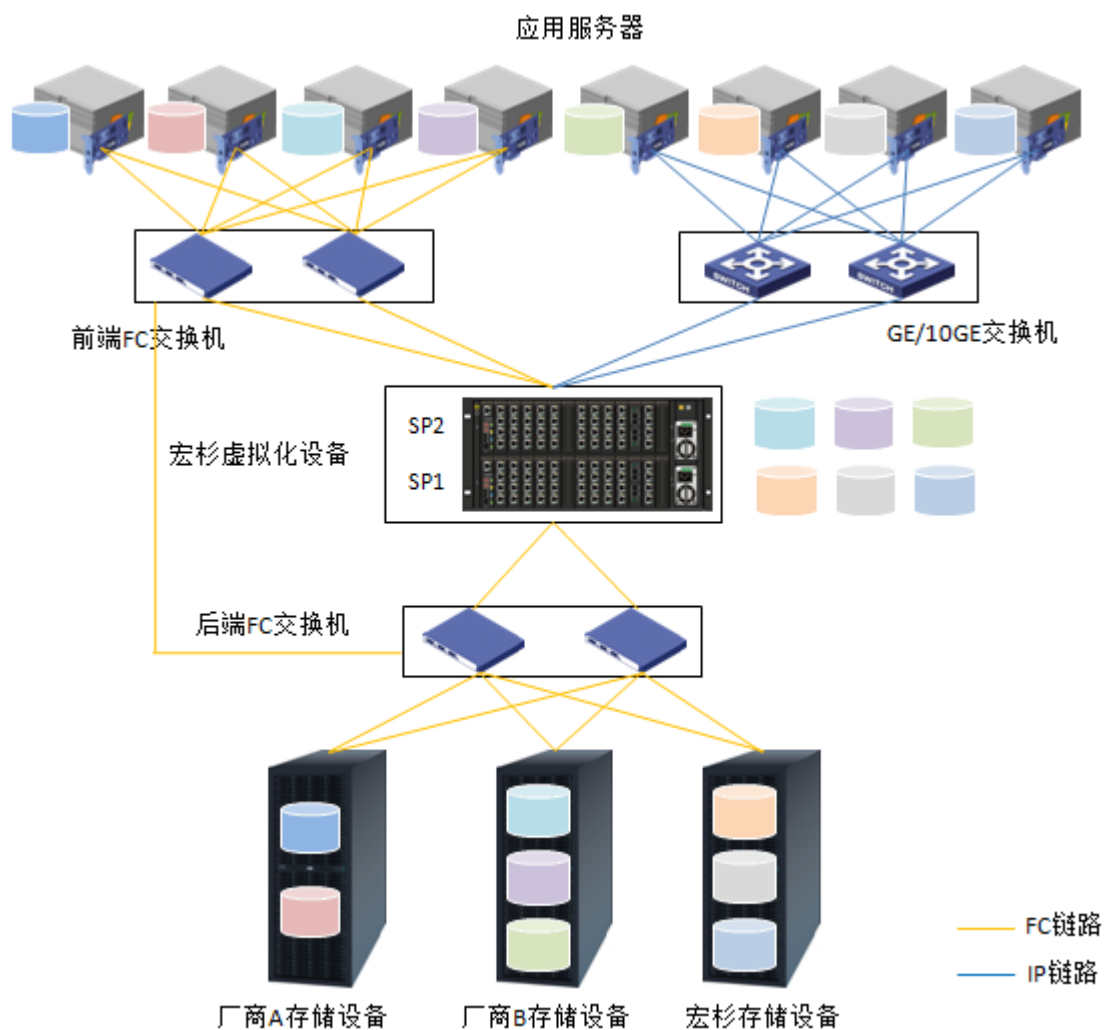
图4-3 宏杉虚拟化设备（管理部分资源）组网图
